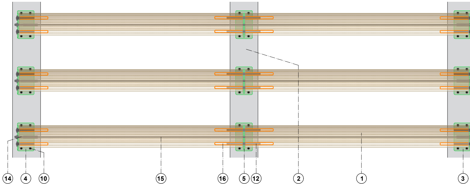
HORIZONTAL SECTION SCALE: 1/8
